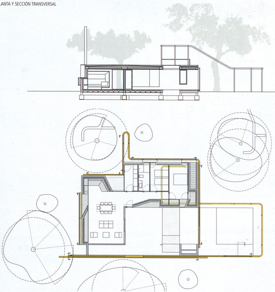
PLANTA Y SECCIÓN TRANSVERSAL
